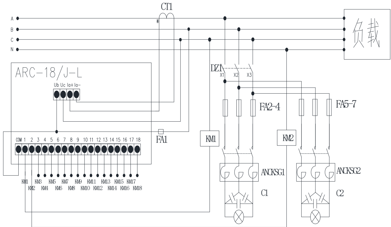
5.2.2.9 配专用接触器的共补接线图（380V）
