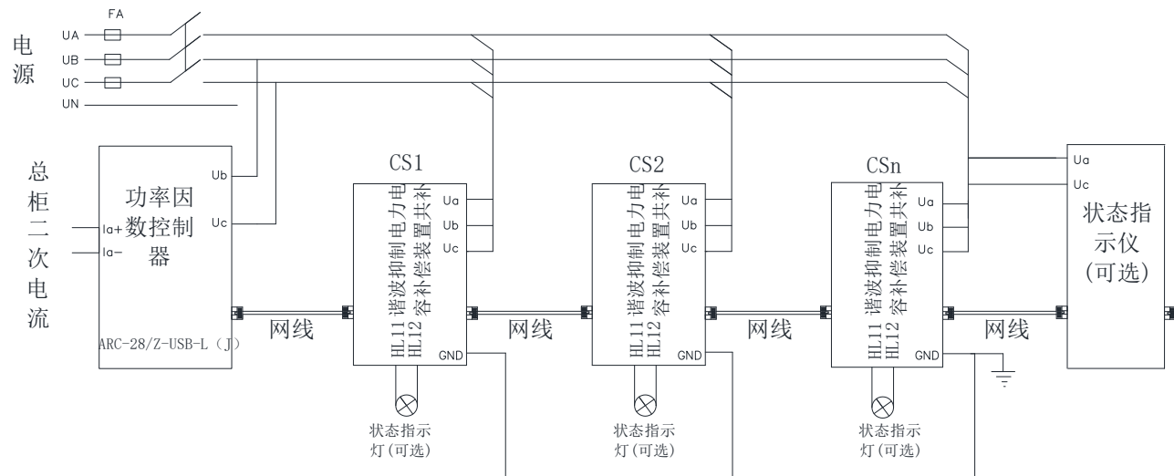
共补接线图（380V 控制器）：
