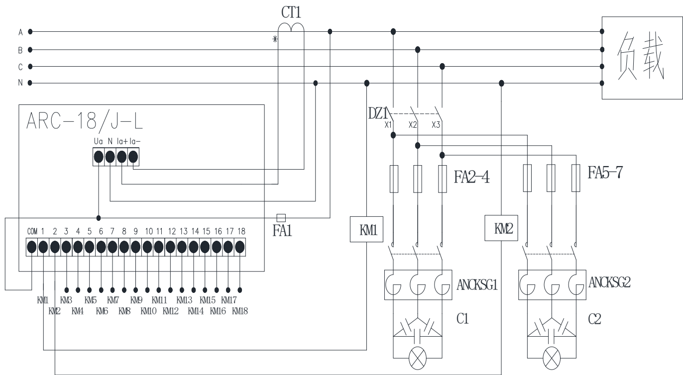
5.2.2.8 配专用接触器的共补接线图（220V）
